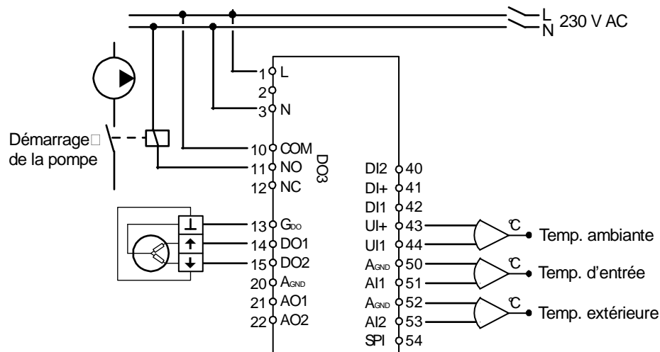
Schéma de câblage pour le mode de régulation n°4
