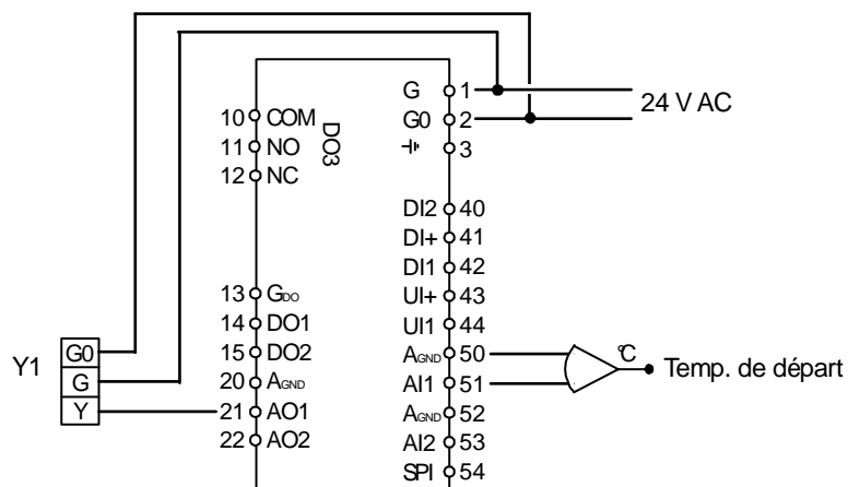
Schéma de câblage pour le mode de régulation 5
